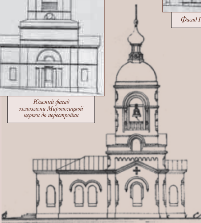
Окончательно утверждённый в 1865 году проект колокольни с церковью
